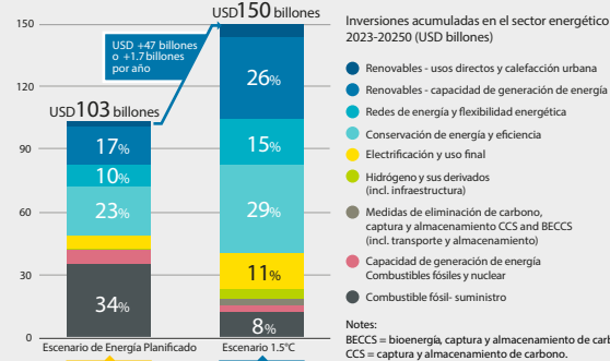
Figure 3.1, Inversión global por vía tecnológica: Escenario Energético Planificado y Escenario 1,5°C, 2023-2050
