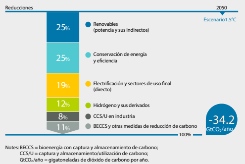
Figura 1.5, Reducción de las emisiones de dióxido de carbono en un escenario de 1,5°C en 2050
